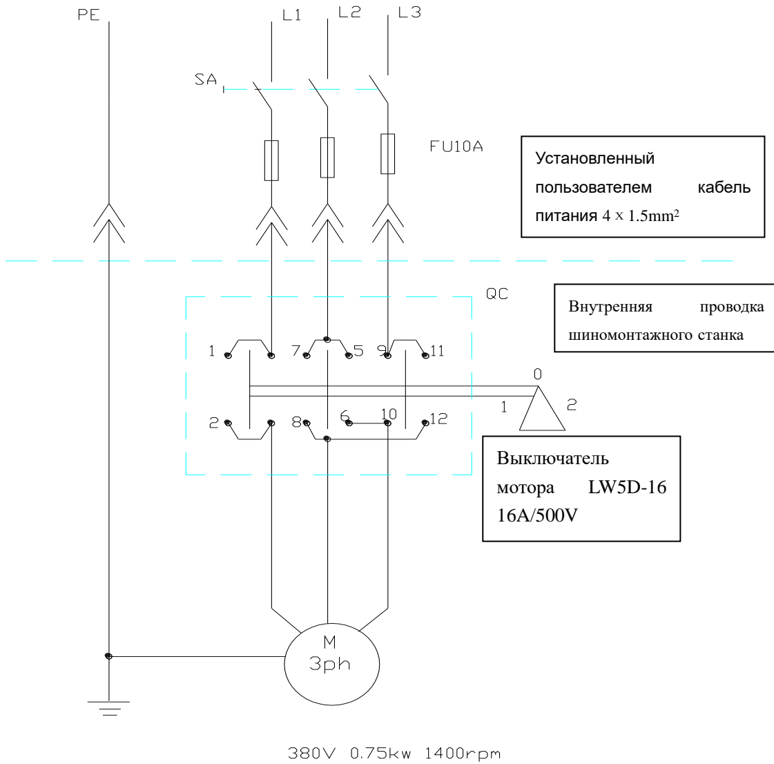
Схема подключения шиномонтажного станка с 3 фазным двигателем 380В
