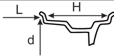
Рисунок 5.4 – Размеры диска при традиционном вводе
