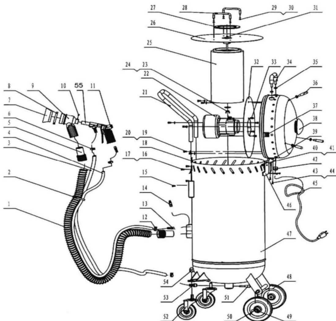
Рис. 1. Устройство изделия.
